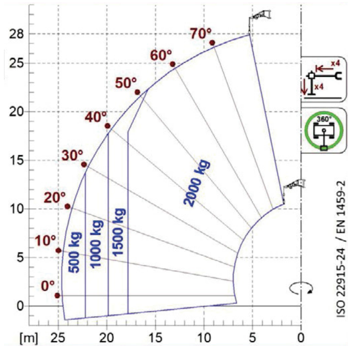
Гусек с лебедкой
