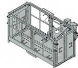
Платформа для персонала раздвижная, поворотная \pm 90^\circ
